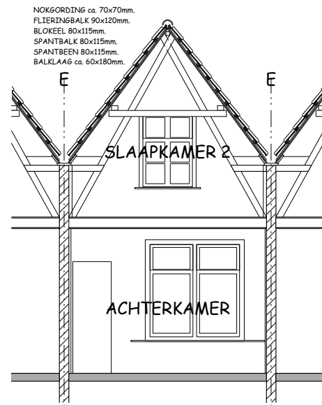
DWARSDOORSNEDE
