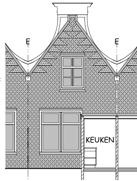
ACHTERGEVEL
