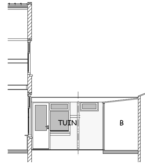
LINKER ZIJGEVEL
